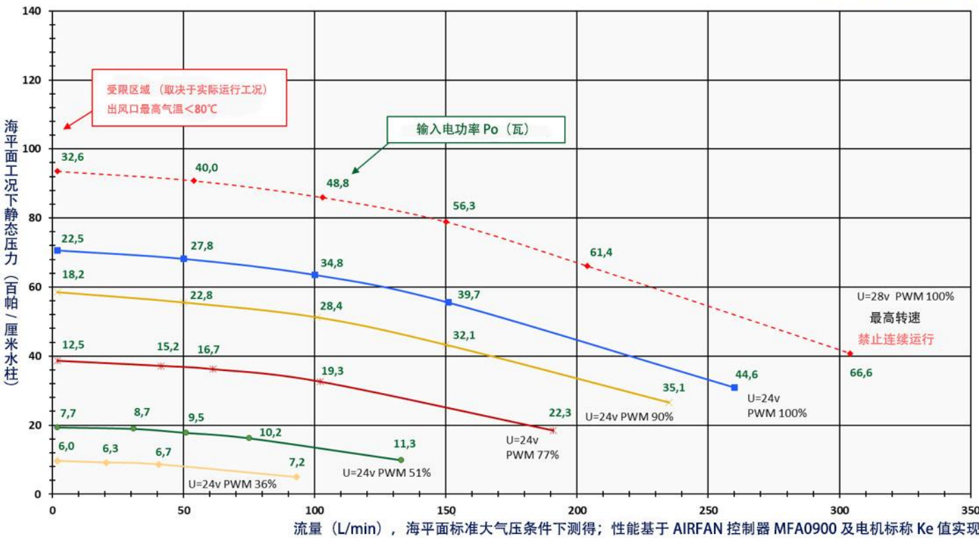
MFA0208型涡轮
